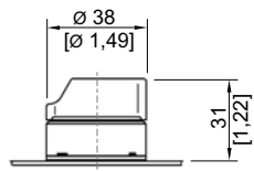
8003/...-726 rotary actuator
